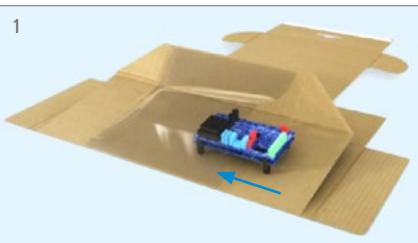
Packgut unter Folie legen
